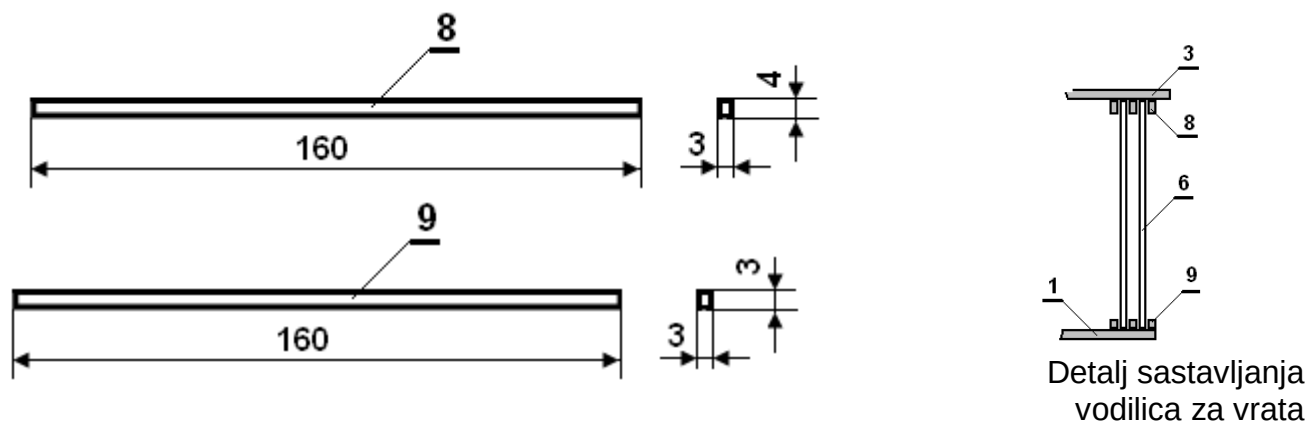
Sastavni crtež modela komode
