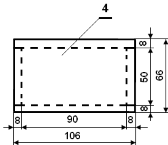
Sastavni crtež ormarića za cipele
